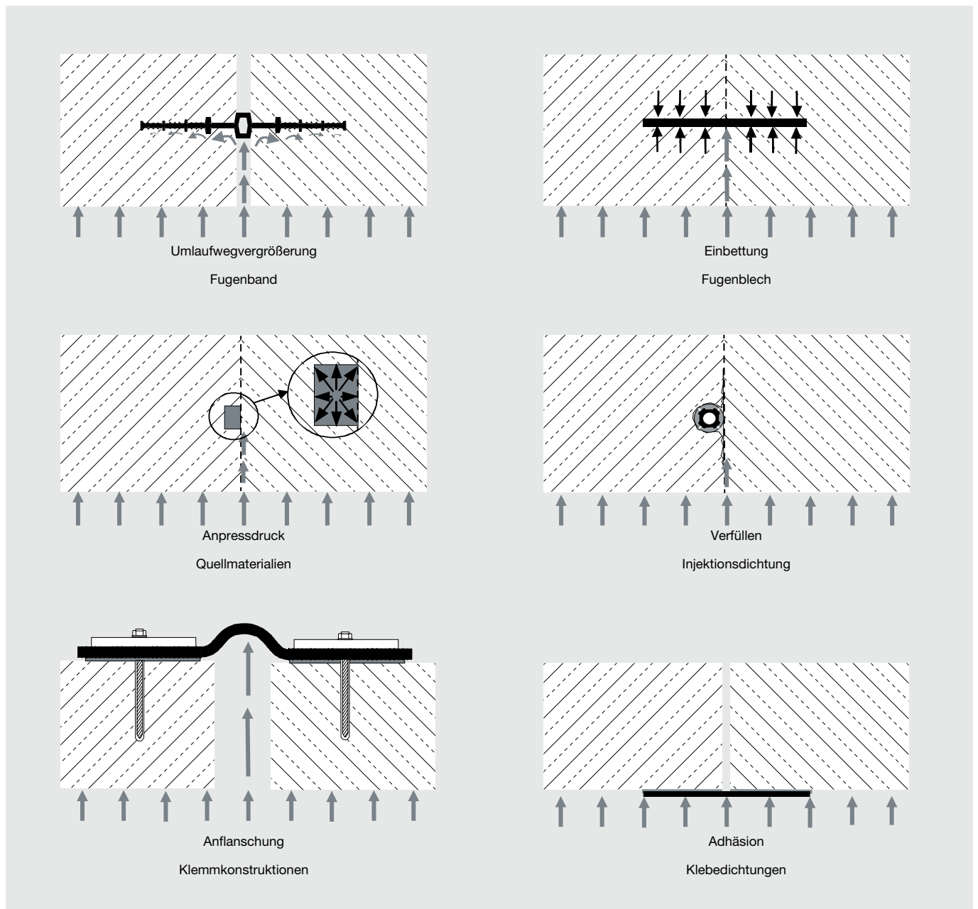
Bild 1: Abdichtungsprinzipien
